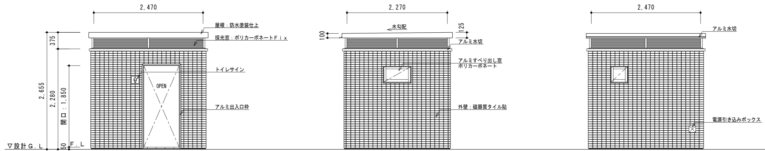
正面図 S = 1 / 5 0
