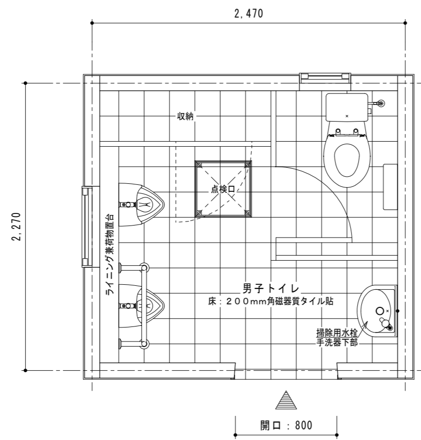
平面図 S = 1 / 3 0
