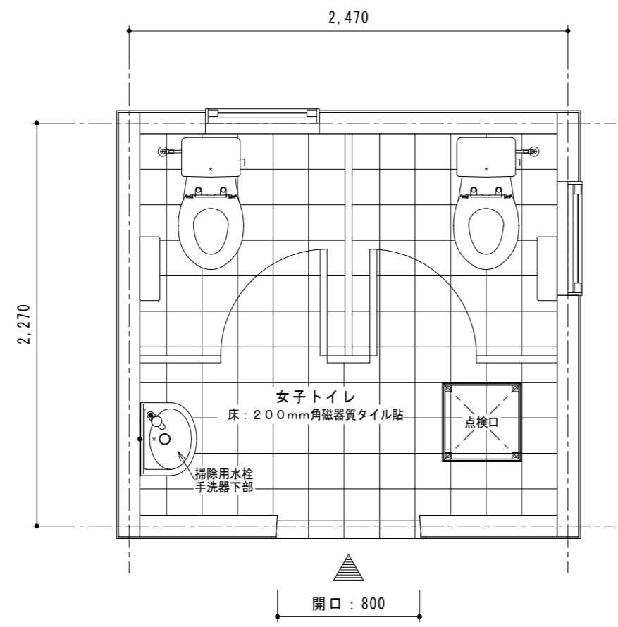
平面図 S = 1 / 3 0
