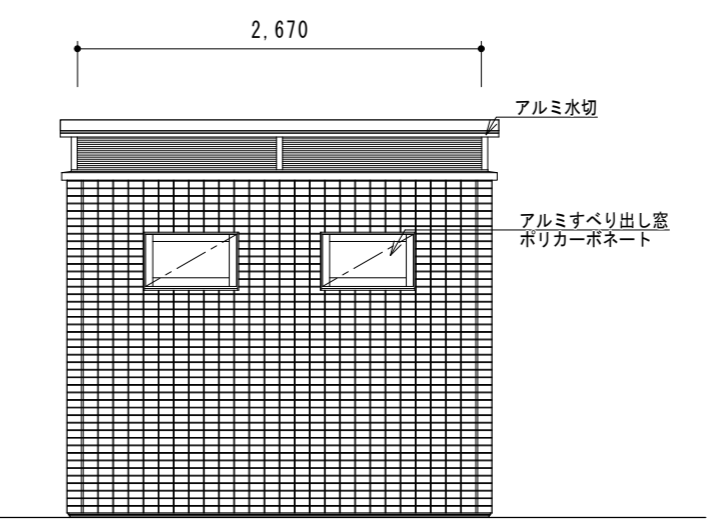
背面図 S = 1 / 5 0
