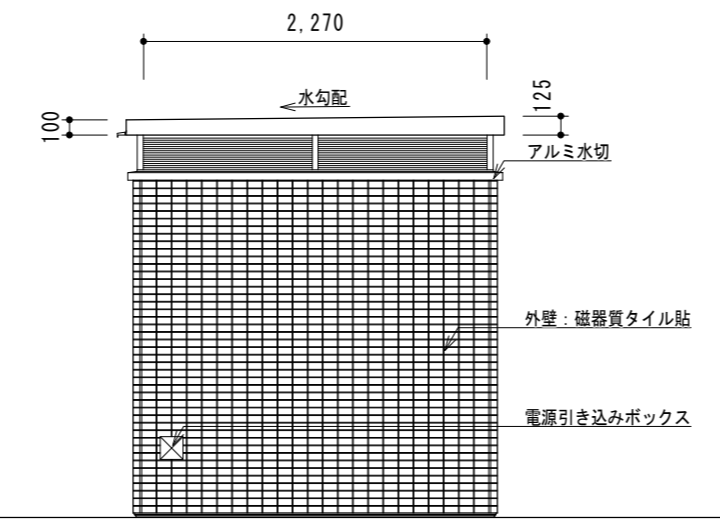
側面図 S = 1 / 5 0
