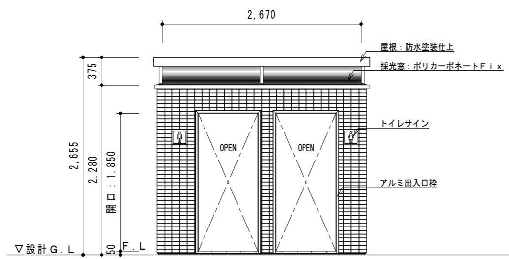
正面図 S = 1 / 5 0
