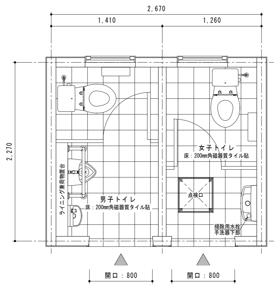
平面図 S = 1 / 3 0
