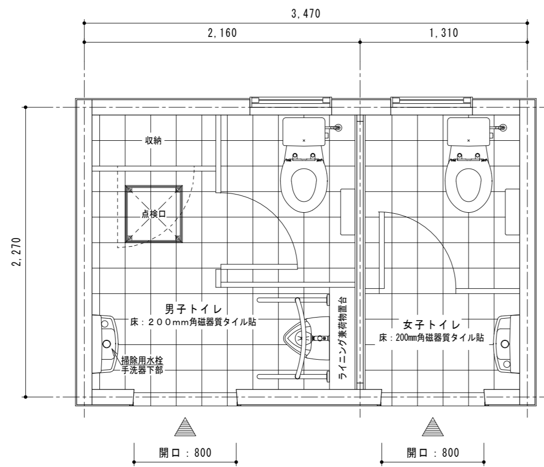
平面図 S = 1 / 3 0
