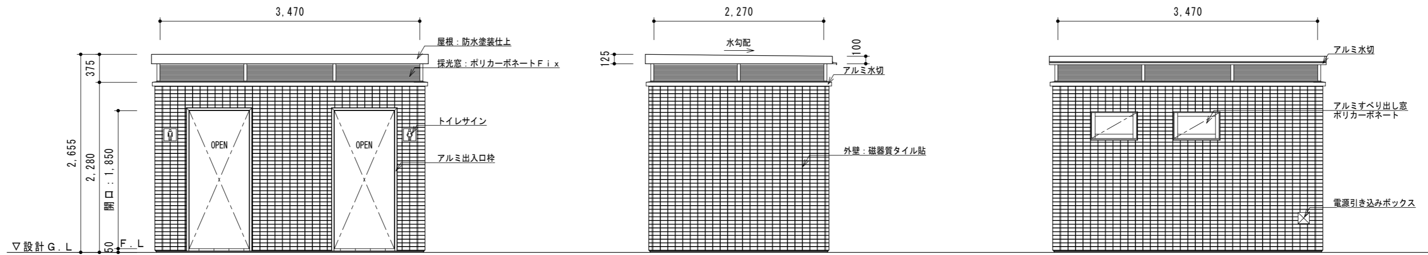
正面図 S = 1 / 5 0
