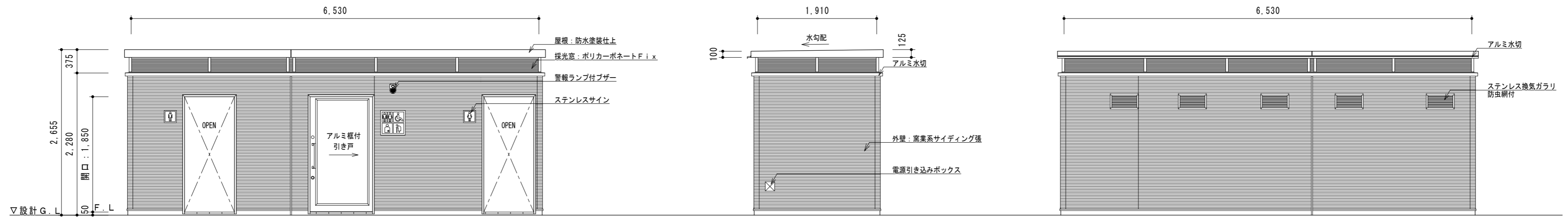
正面図 S = 1 / 5 0
