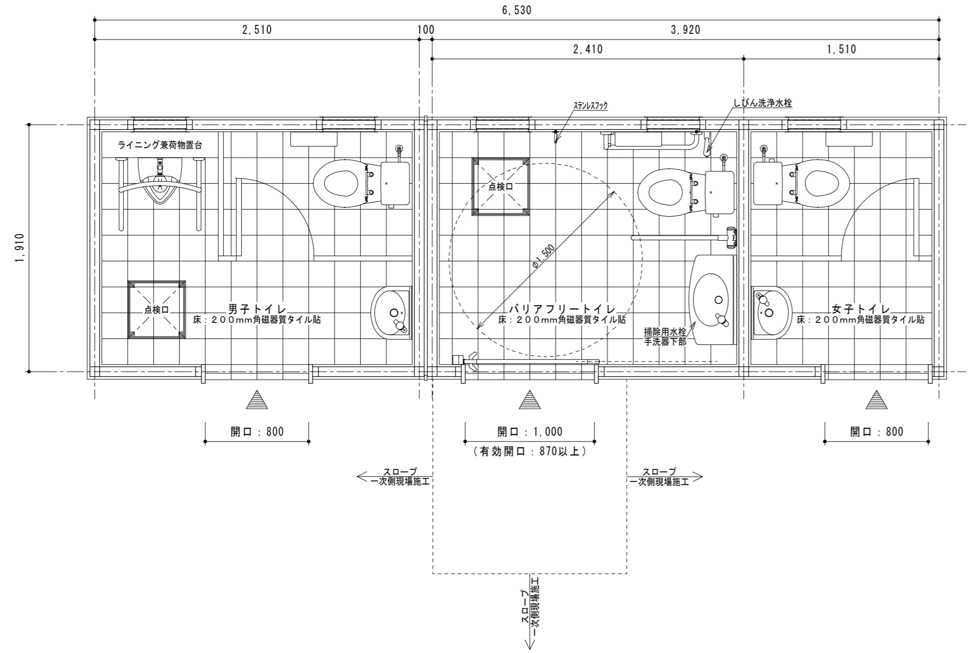
平面図 S = 1 / 3 0
