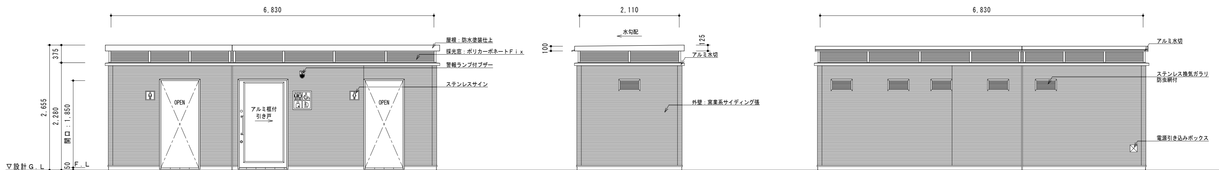
正面図 S = 1 / 5 0
