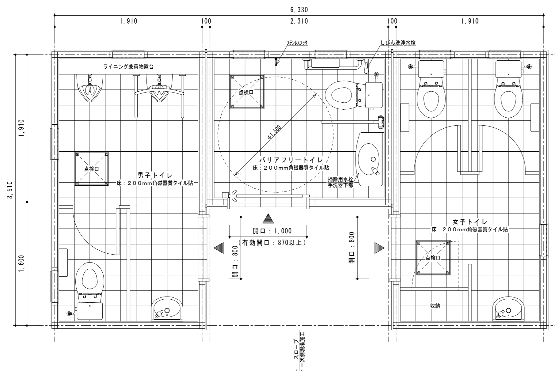
平面図 S = 1 / 3 0
